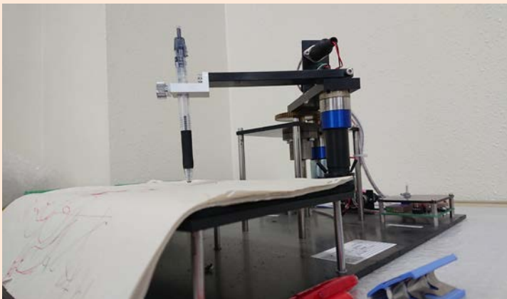
ロボットアーム
