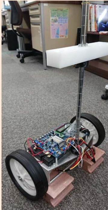
2輪型倒立振り子
